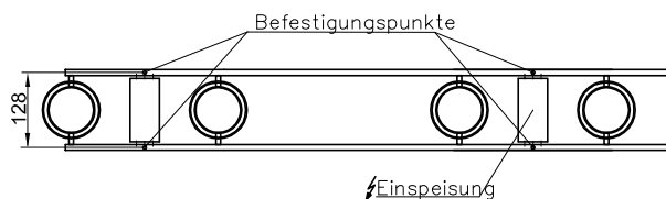
Draufsicht
