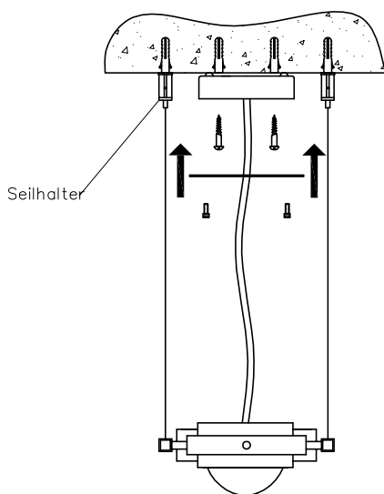
Seitenansicht
