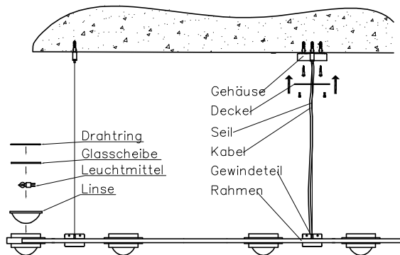
Frontansicht
